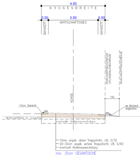
Abbildung 3: Standardausgestaltung Begleitweg
